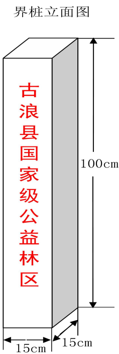
图一 界桩示意图
