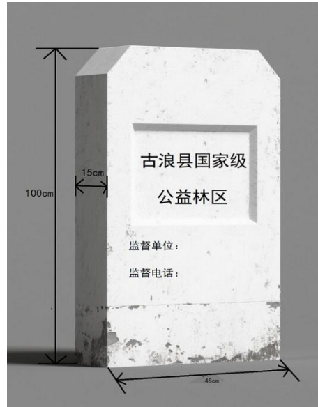
图二 界碑示意图
