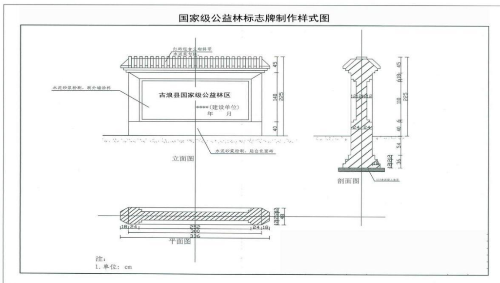
图三 标志牌示意图
