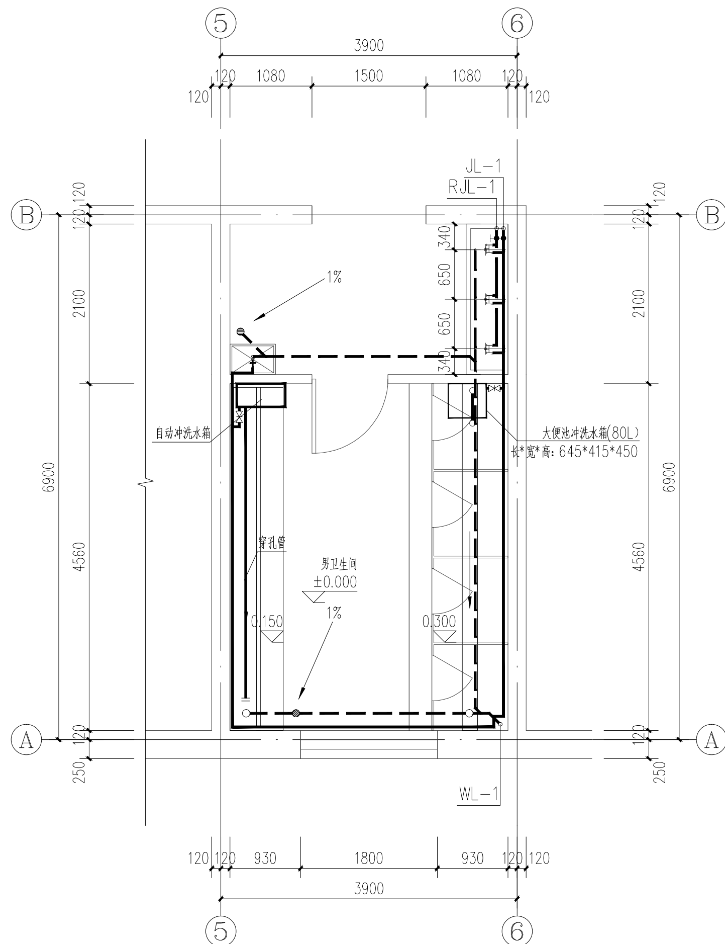
卫生间给排水详图 1:50
