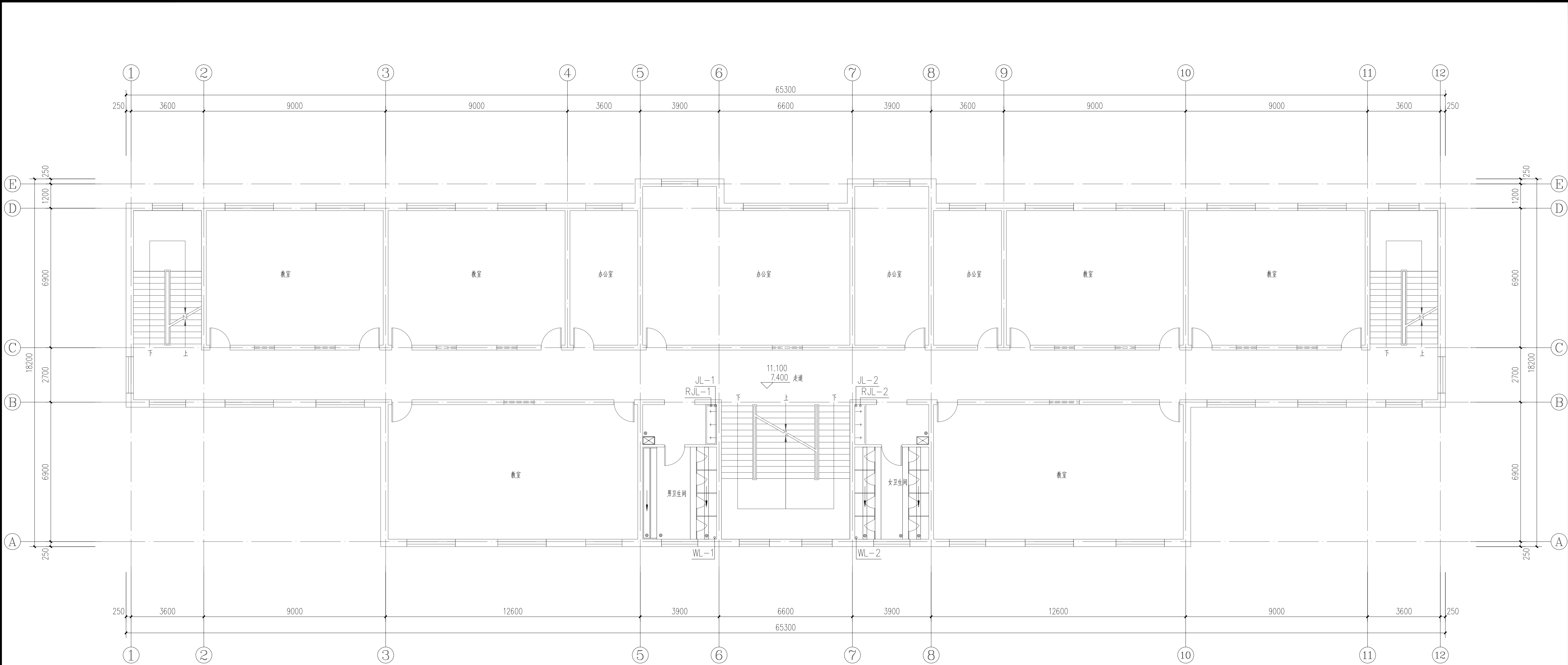
三-四层给排水平面图 1:100
