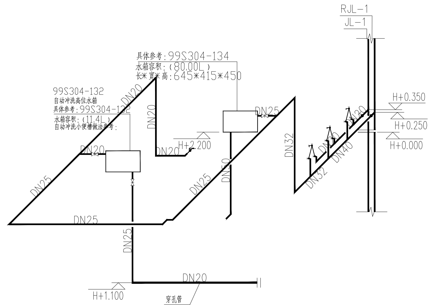
给水系统图 1:50
