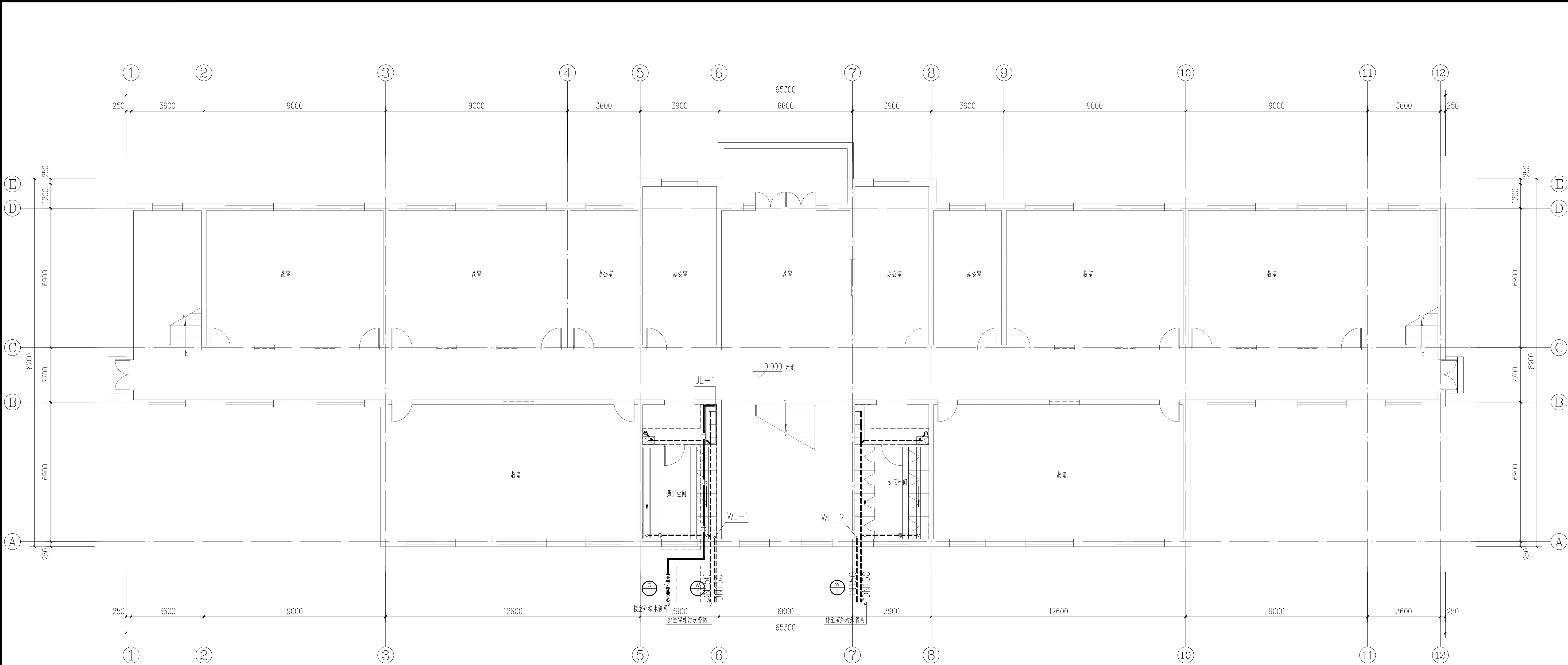
一层地沟给排水平面图 1:100
