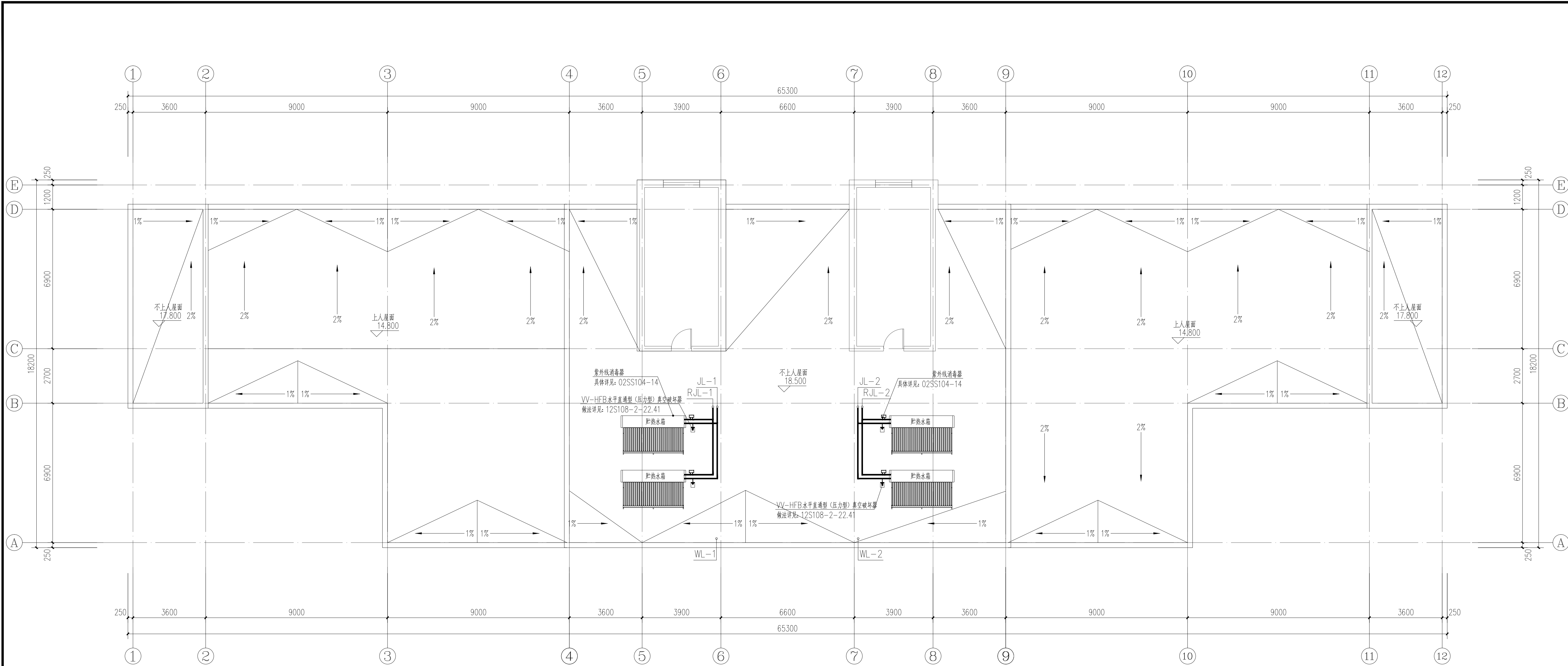
屋顶给排水平面图 1:100
