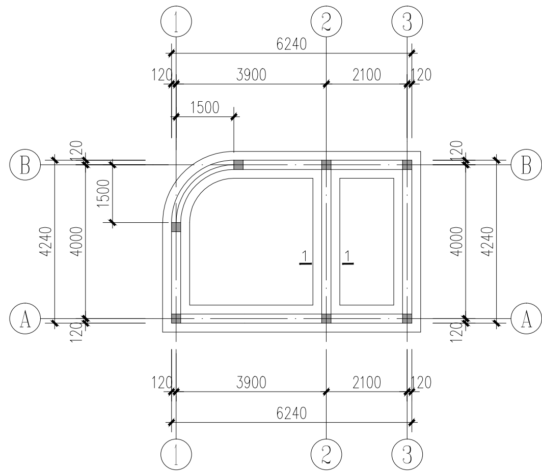
基础平面布置图
