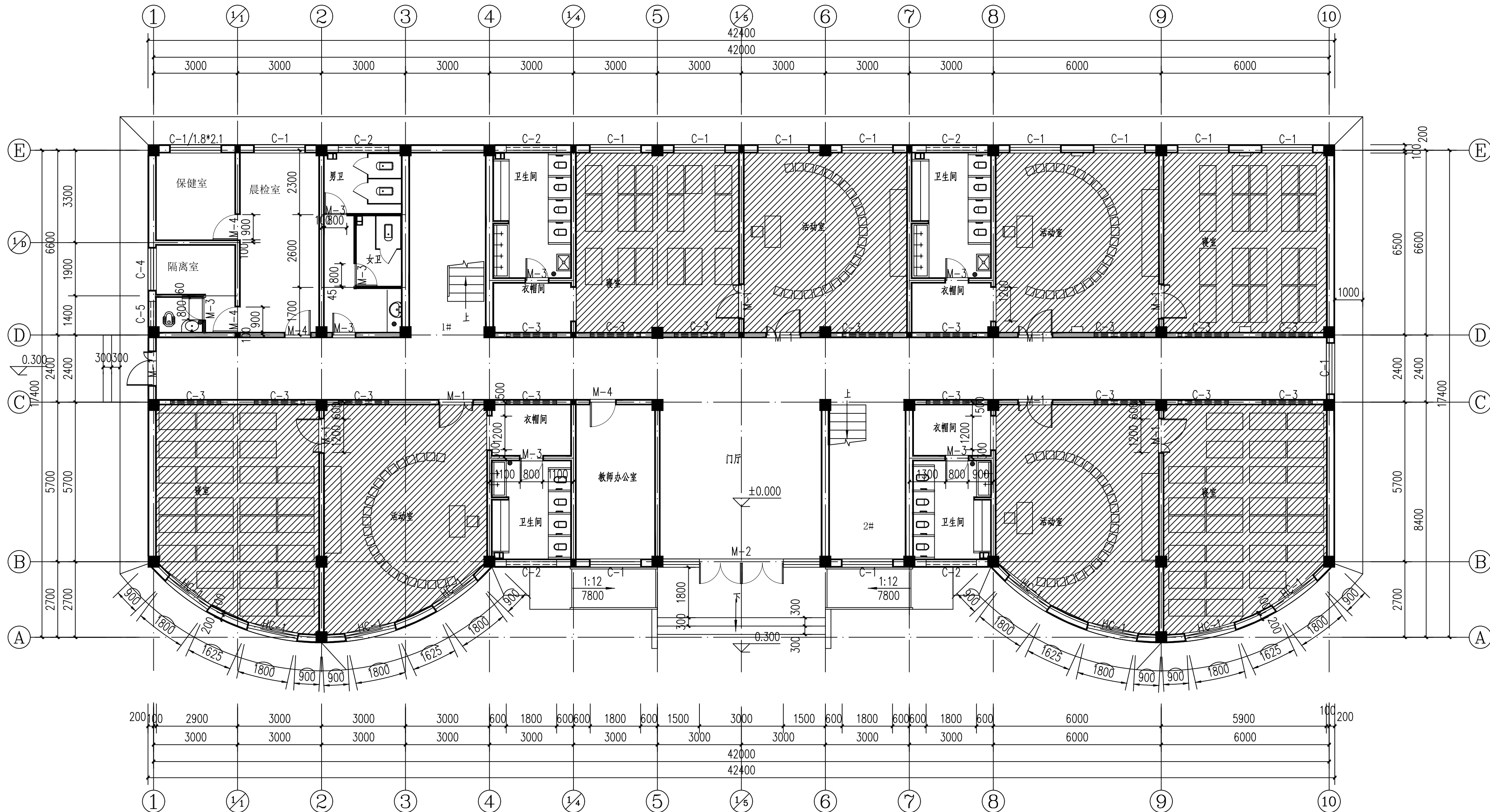
一层平面图 1:100
