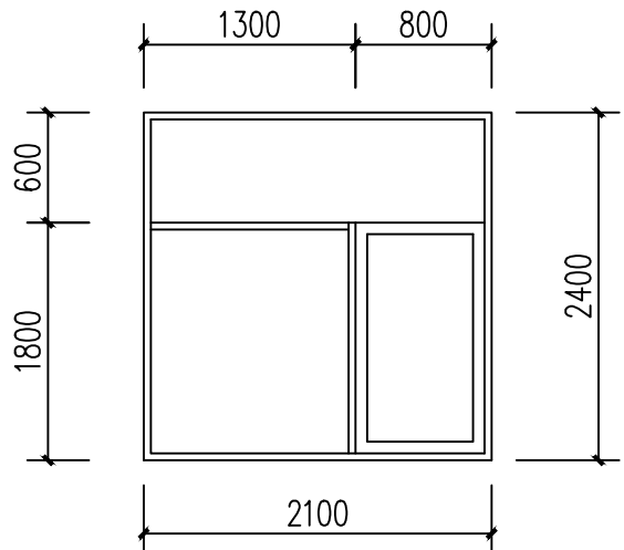
C2124立面图 1:50
