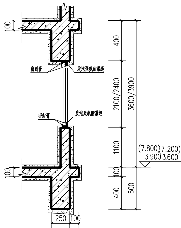
走廊封闭做法
