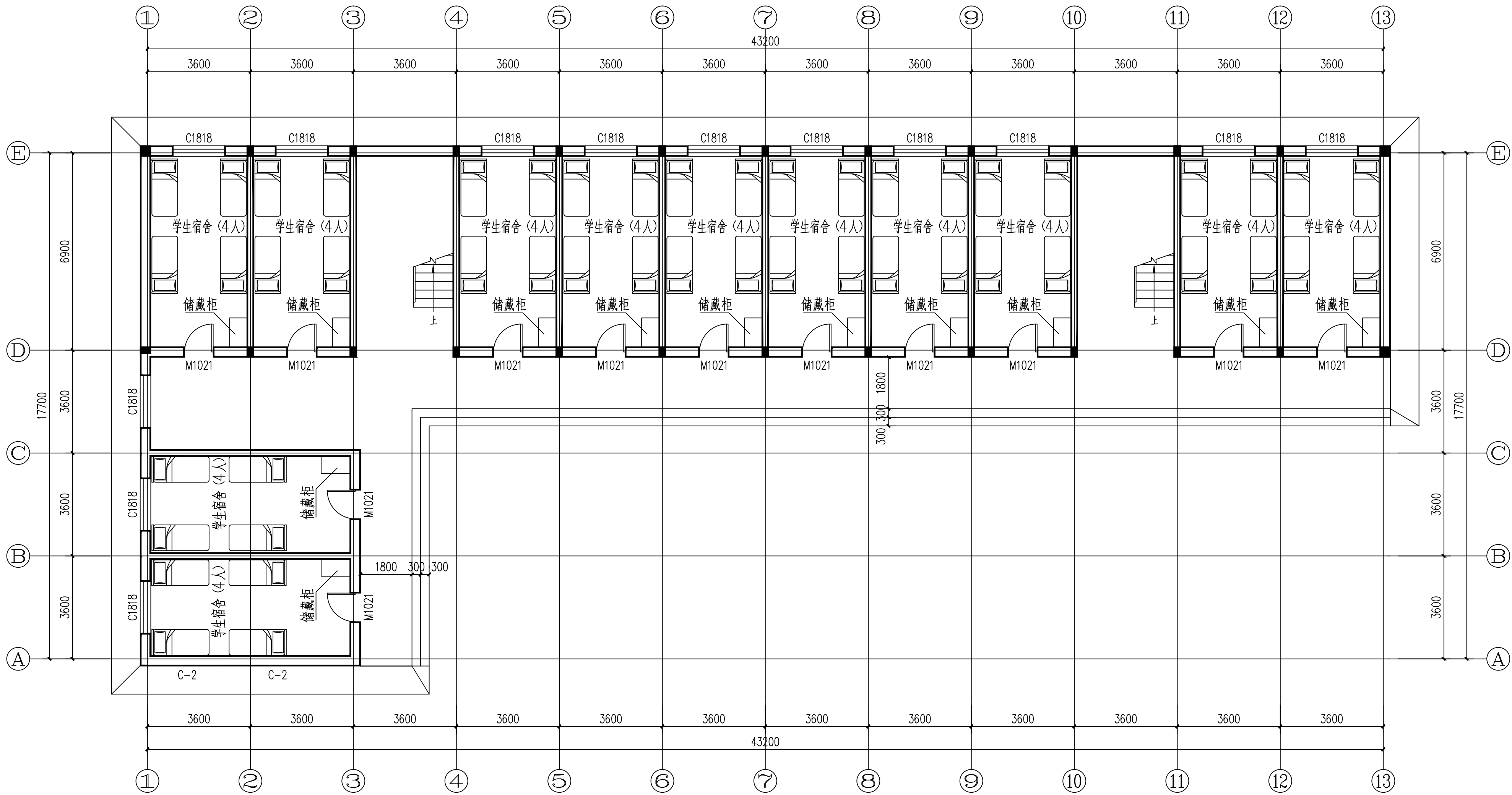
一层平面图 1:100
