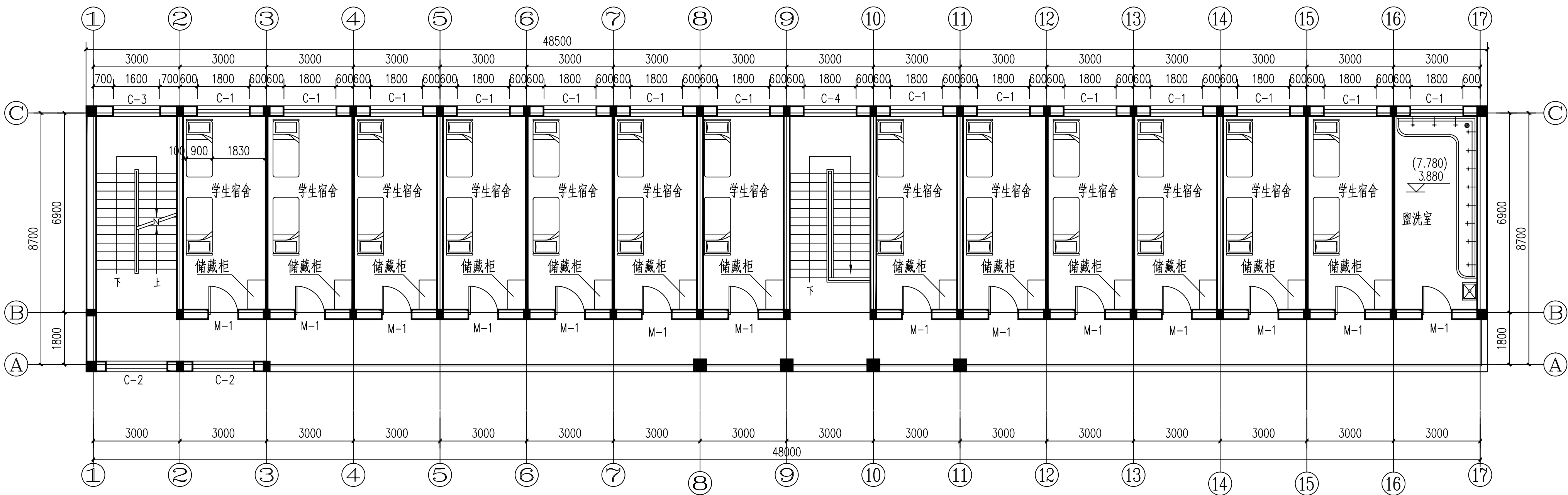
二-三层平面图 1:100
