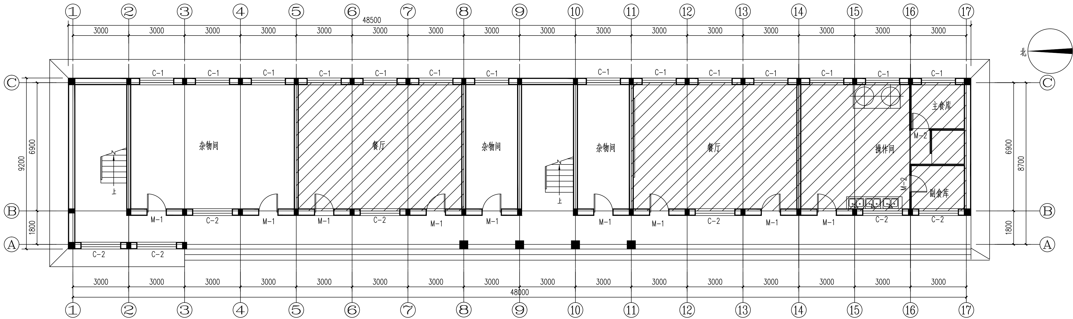
一层平面图 1:100
