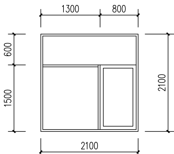
C2121立面图 1:50
