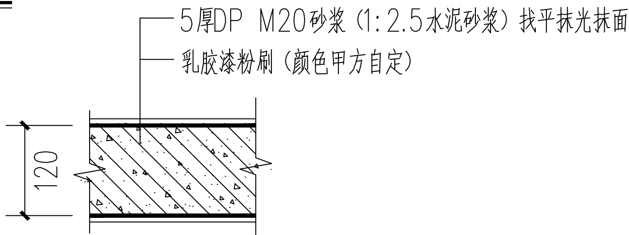
门窗洞口粉刷做法
